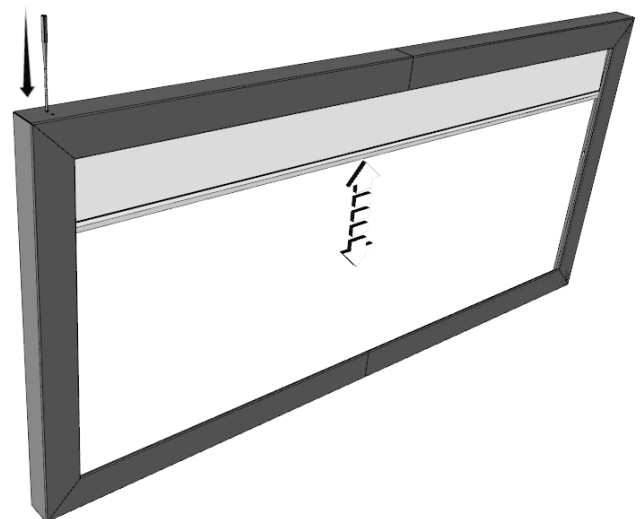
AGUJERO CERCA DE LA PARED REGULACION DE LOS FINALES DE CARRERA ALTO
